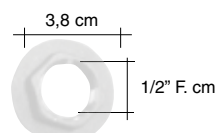
Controdado c/flangia 1/2" F. Hexagon lock nut 1/2" F.
